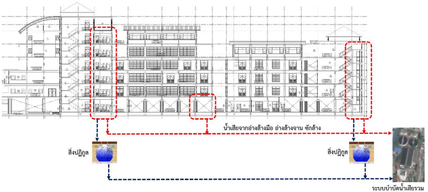
ภาพที่ 4.2.1-3 (1) ผังการจัดการน้ำเสีย คณะสถาปัตยกรรมศาสตร์
